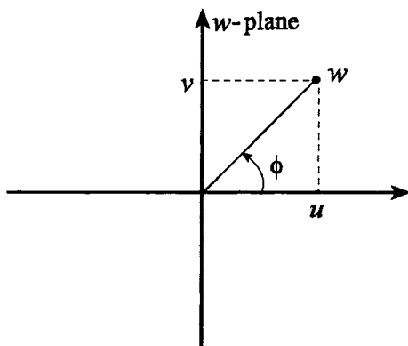
Fig. 12.2 w -plane
