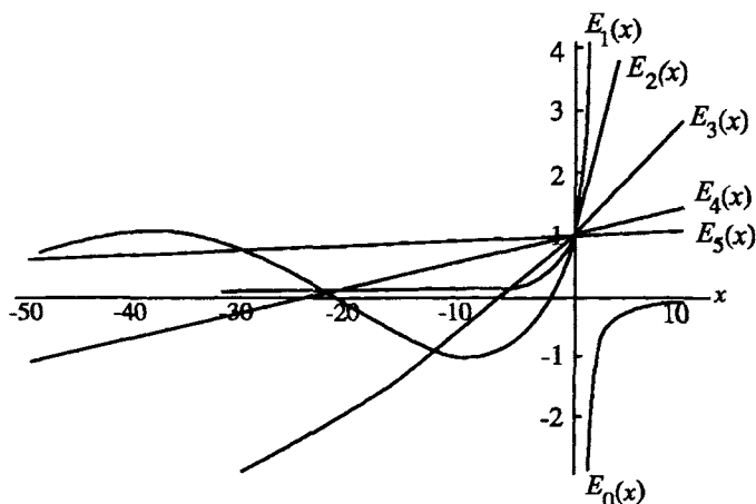
Fig. 14.5 Mittag-Leffler functions
