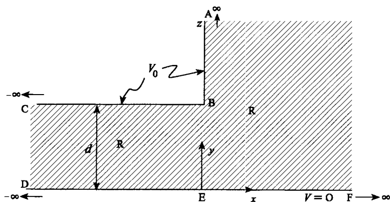
Fig. 12.29 Schwartz-Christoffel transformation
