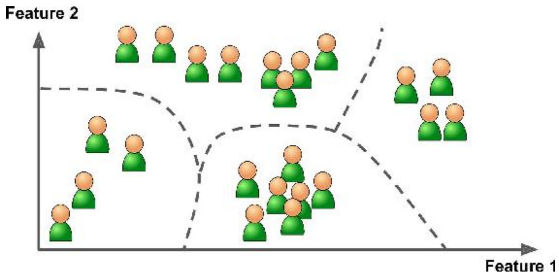
Figure 1-8. Clustering
